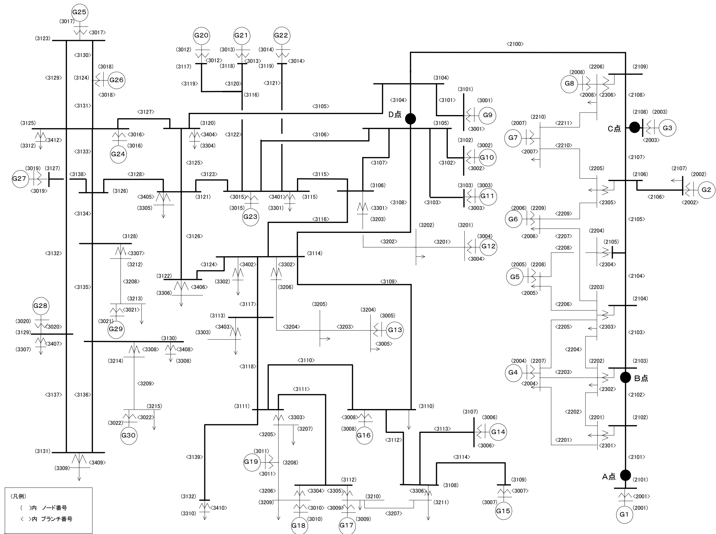
4.15図 電気学会EAST30機系統モデル 系統図(ノード番号、ブランチ番号、事故点含む)
