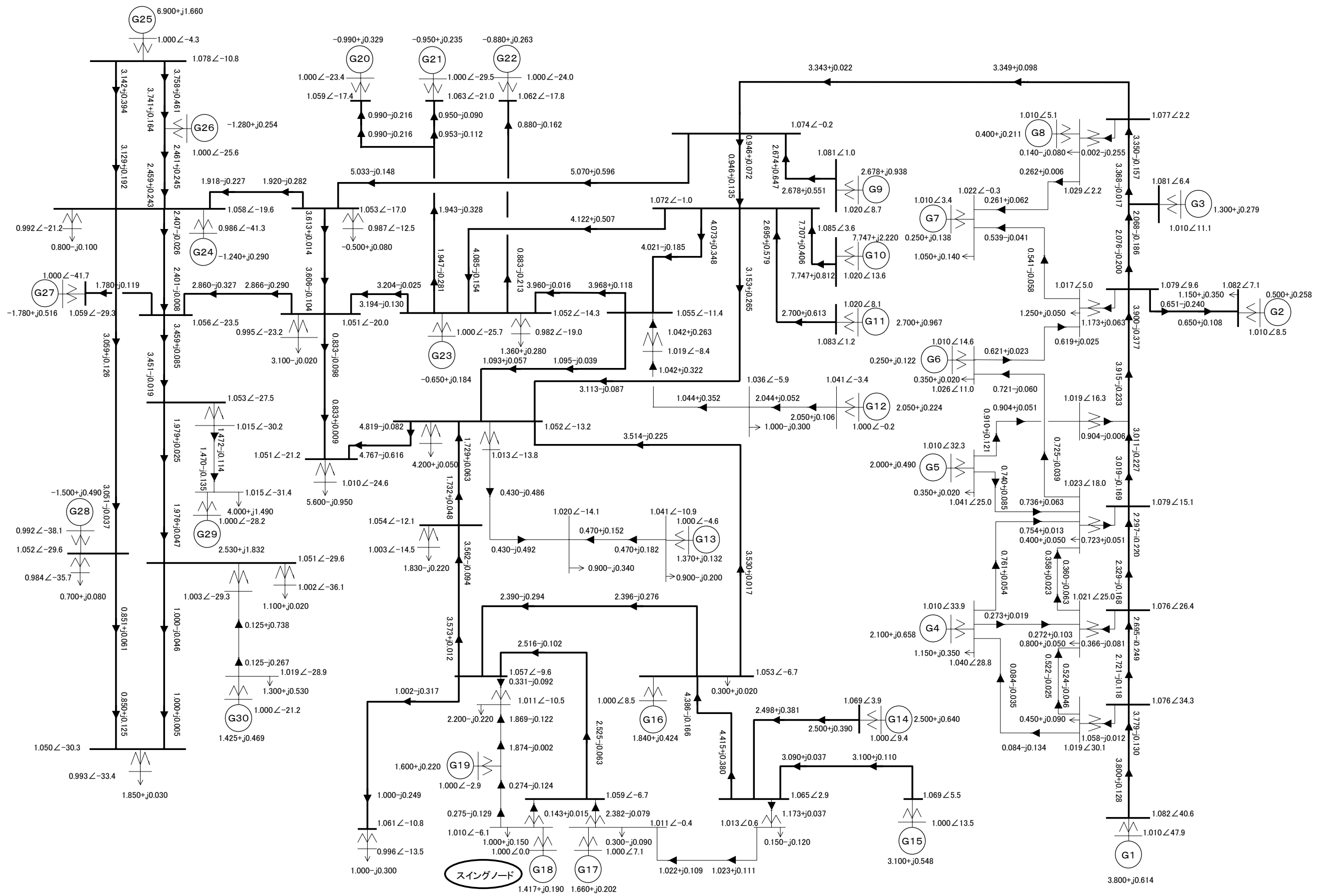
4.17図 (b) 電気学会EAST30機系統モデル 潮流図(夜間断面)
