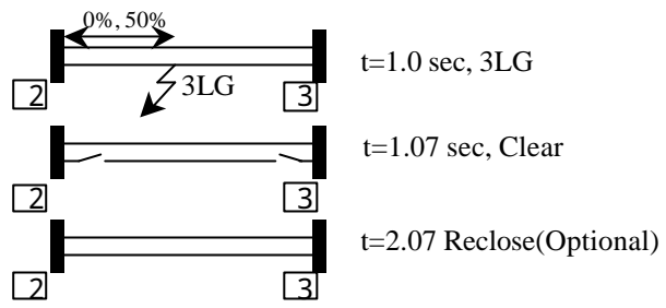
付図 3.3 事故シーケンス
