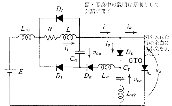
図1 スナバエネルギー回生回路
